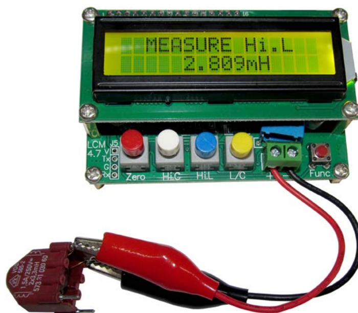
Měření indukčnosti – nezáleží na polaritě
